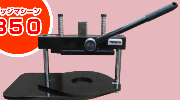
■サイズ(mm) : L620×W400×H345(レバー除く) ※アタッチメント 158、250、350 が取付可能です
